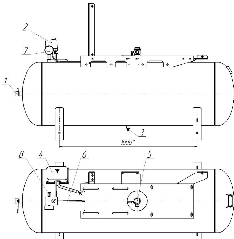
Рис.10 Ресивер, модель С416М1, С416М1-01, С416М1-02 1-вентиль раздаточный; 2- реле давления; 3-пробка сливная; 4-коробка клеммная; 5-обратный клапан; 6-разгрузочная трубка; 7-манометр; 8-клапан предохранительный.
