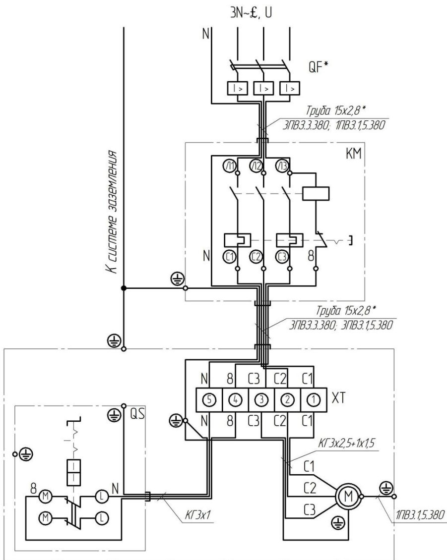
Рис.18 Схема электрическая принципиальная и соединений компрессора, модель C416M1, C416M1-01
