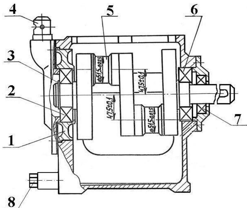
Рис.5 Картер:
