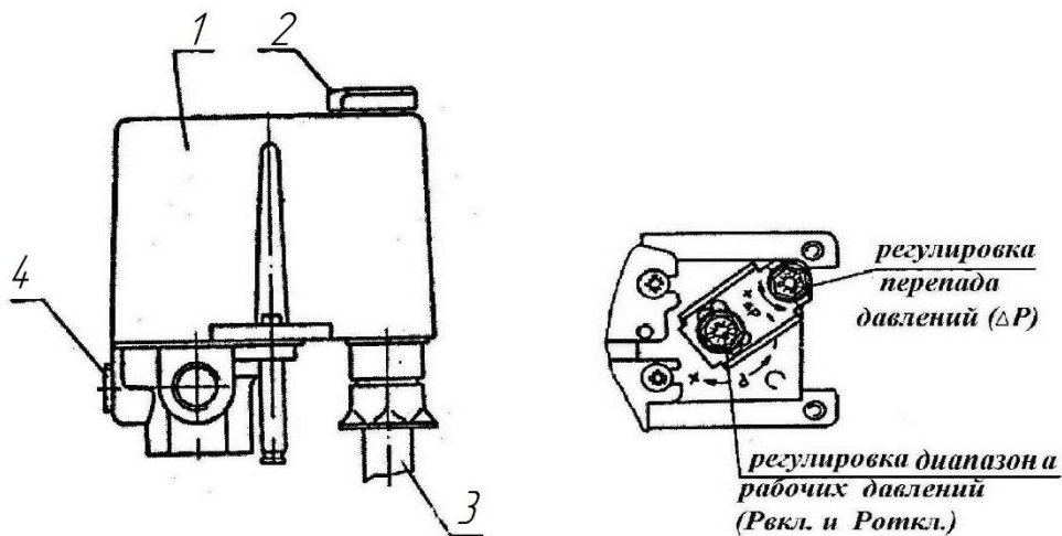
Рис. 12 Реле давления MDR 3/11, MDR 3/16 1- кожух, 2- переключатель, 3- кабель, 4- заглушка.
