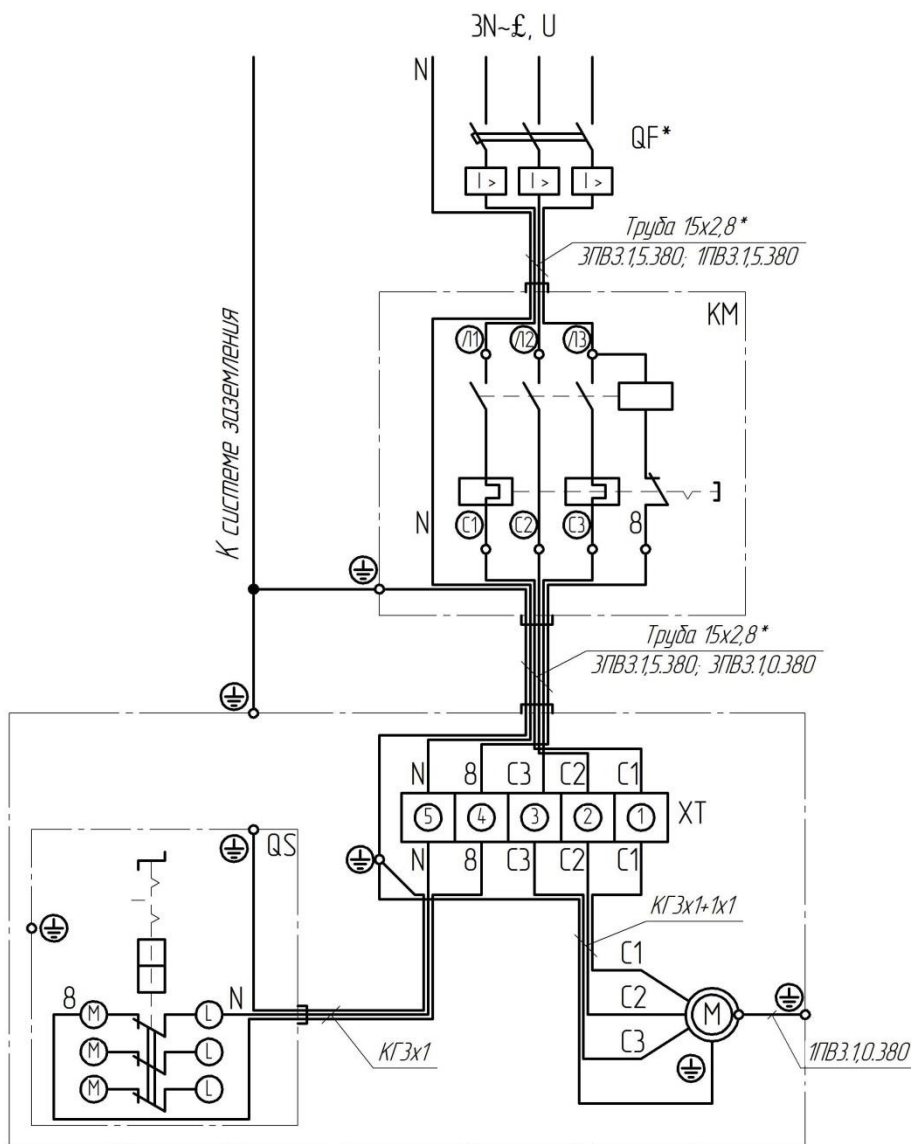
Рис.19 Схема электрическая принципиальная и соединений компрессора, модель C415M1-02
