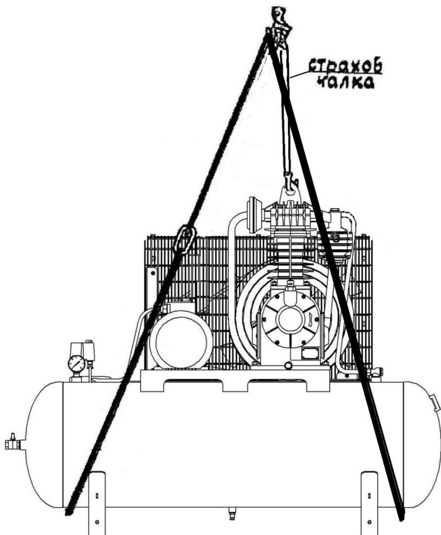
Рис.21 Схема строповки установки компрессорной модель С415М1, С415М1-01, С415М1-02
