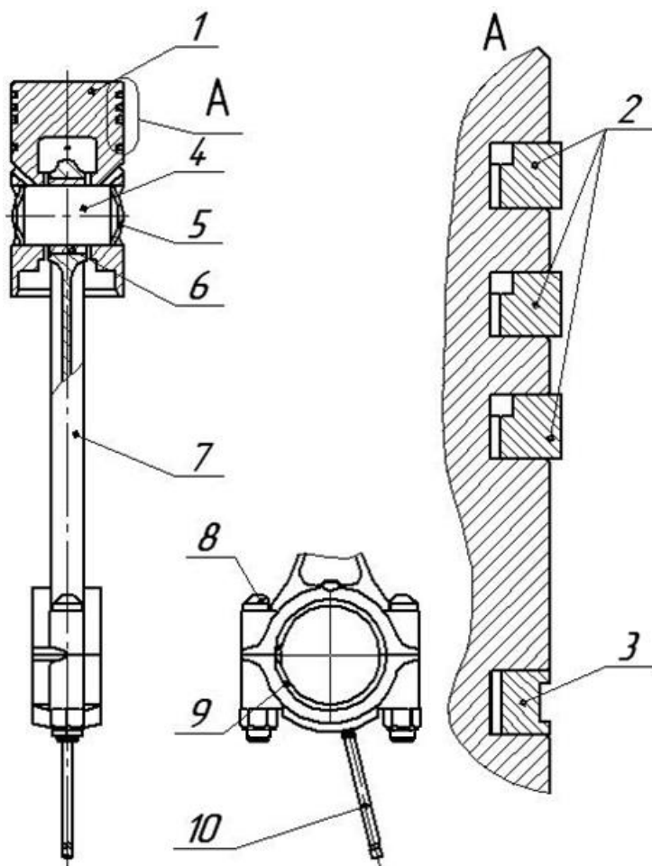
Рис.7 Поршень цилиндра высокого давления:
