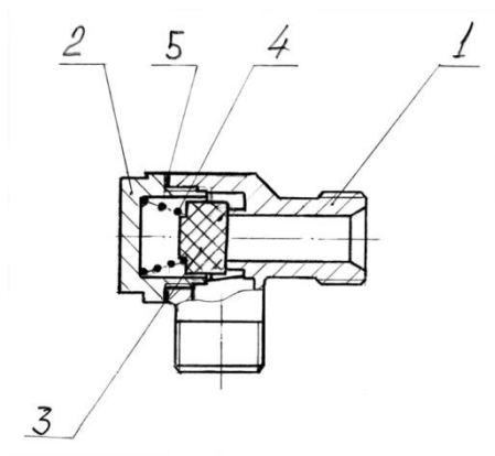
Рис.14 Клапан обратный
