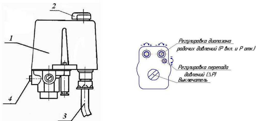
Рис.11 Реле давления MDR 2/11 1-кожух; 2-переключатель; 3-кабель; 4-заглушка.
