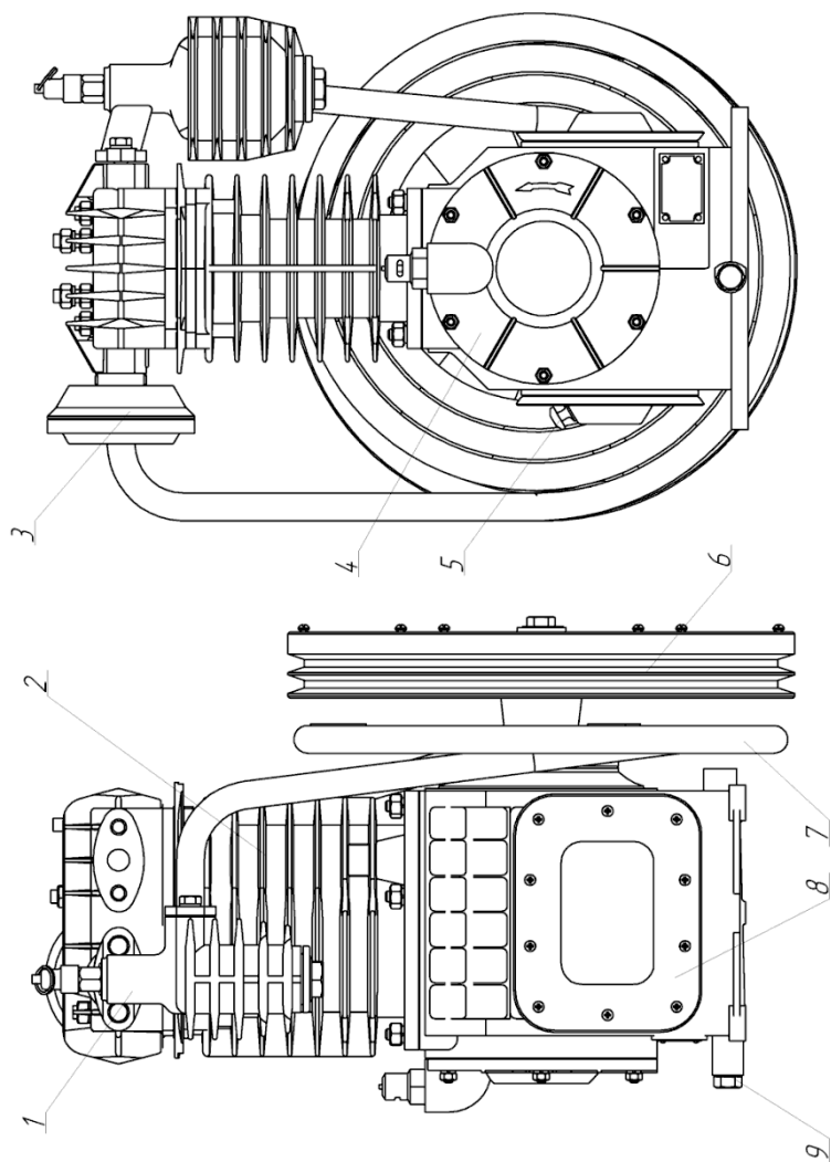
Рис. 3 Головка компрессорная, модель S415M
