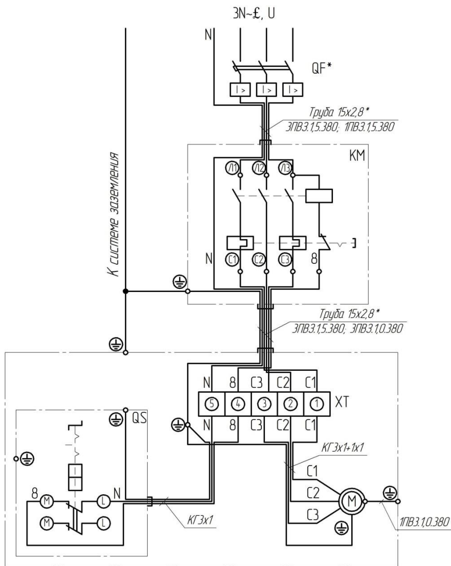
Рис.17 Схема электрическая принципиальная и соединений компрессора, модель C415M1, C415M1-01
