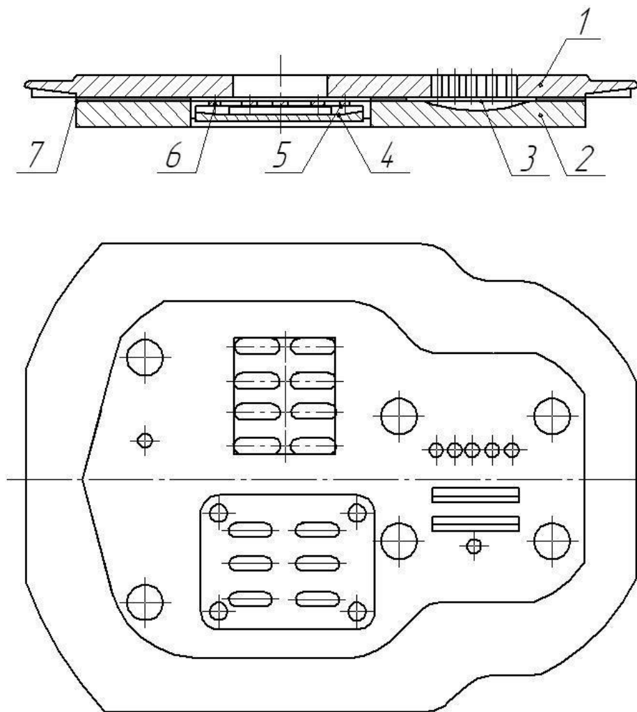
Рис.8 Блок клапанный:
