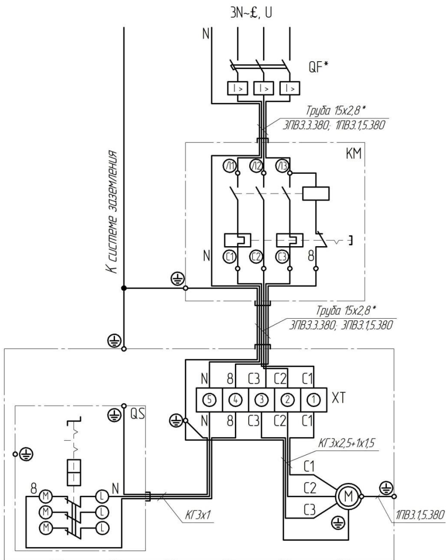
Рис.20 Схема электрическая принципиальная и соединений компрессора, модель C416M1-02
