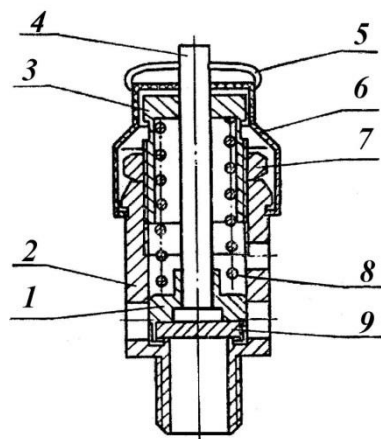
Рис.13 Клапан предохранительный
