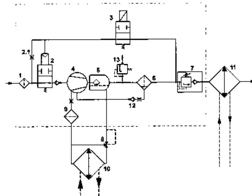
Рисунок 14. Принципиальная пневмогидравлическая схема винтового модуля (с электромагнитным управлением).
