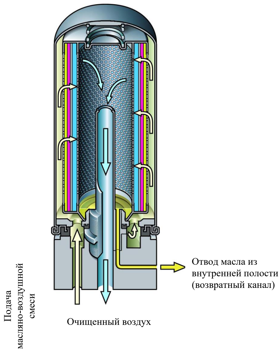
Рисунок 7. Картридж сепаратора.
