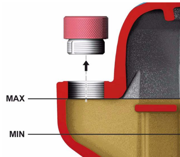
Горловина заливная винтового модуля EVO3-NK
