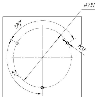
Схема расположения фундаментных болтов
