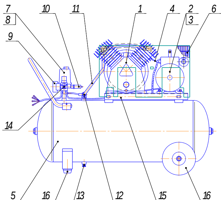
Рисунок 7 - Общий вид компрессоров СБ4/С-100.LB30, СБ4/С-100.LB30А
