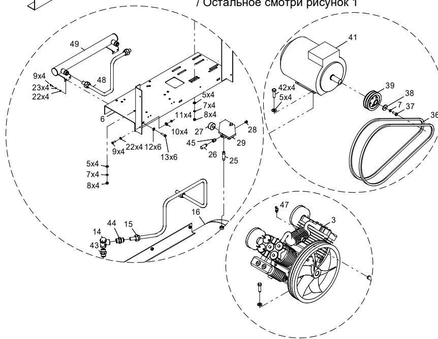
Figure 3 / Abbildung 3 / Рисунок 3 CB4/F-500.LT100/16-7,5 SB4/F-500.LT100/15-7,5 Else see Figure 1 / Else siehe Abbildung 1 / Остальное смотри рисунок 1
