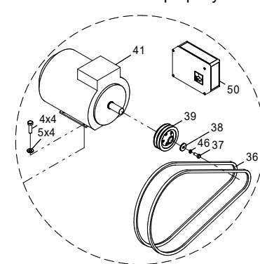
Figure 4 / Abbildung 4 / Рисунок 4 CБ4/Ф-500.LT100/16 SB4/F-500.LT100/15 Else see Figure 3 / Else siehe Abbildung 3 / Остальное смотри рисунок 3
