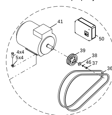
Figure 4 / Abbildung 4 / Рисунок 4 СБ4/Ф-500.LT100/16 SB4/F-500.LT100/15 Else see Figure 3 / Else siehe Abbildung 3 / Остальное смотри рисунок 3
