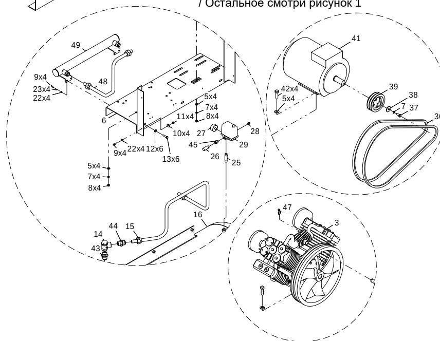
Figure 3 / Abbildung 3 / Рисунок 3 СБ4/Ф-500.LT100/16-7,5 SB4/F-500.LT100/15-7,5 Else see Figure 1 / Else siehe Abbildung 1 / Остальное смотри рисунок 1
