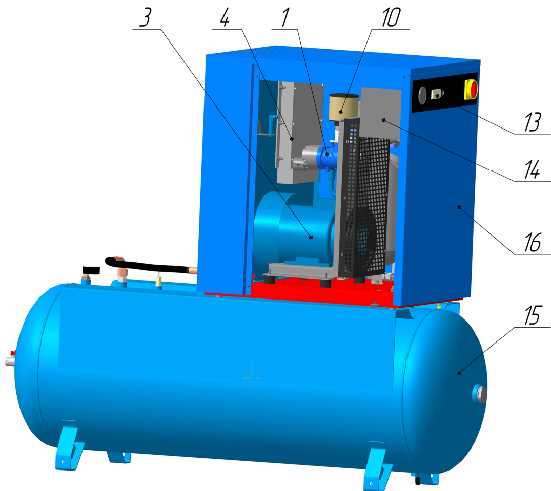
Рисунок 4 – Общий вид компрессорной установки ВК5Т-...-500, ВК7Т-...-500, ВК10Т-...-500
