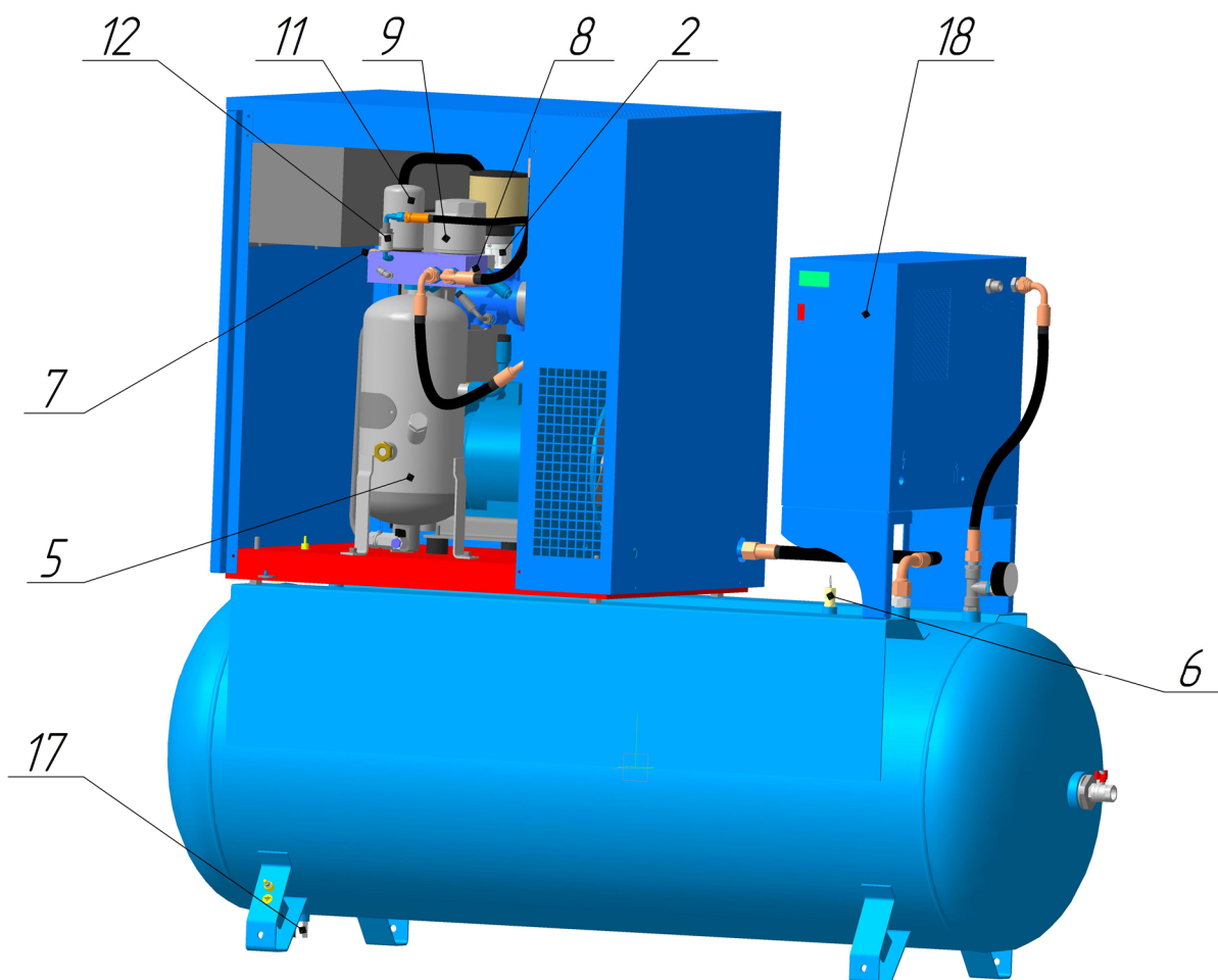
Рисунок 5 – Общий вид компрессорной установки ВК5Т-...-500Д, ВК7Т-...-500Д, ВК10Т-...-500Д
