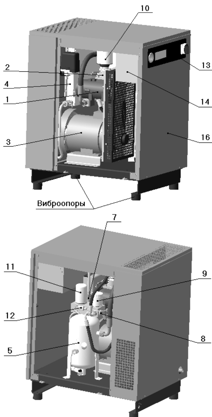
Рисунок 1 – Общий вид компрессорной установки ВК5Т-..., ВК7Т-..., ВК10Т-...
