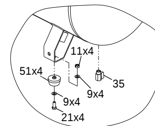
Figure 2 / Abbildung 2 / Рисунок 2 СБ4/Ф-200.ЛБ40 SB4/Ф-200.ЛБ40 Else see Figure 1 / Else siehe Abbildung 1 / Остальное смотри рисунок 1
