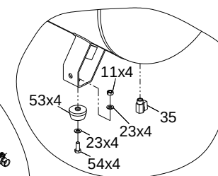
Figure 4 / Abbildung 4 / Рисунок 4 СБ4/Ф-200.LB40 SB4/F-200.LB40 Else see Figure 1 / Else siehe Abbildung 1 / Остальное смотри рисунок 1
