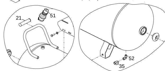
Figure 3 / Abbildung 3 / Рисунок 3 GK 500-3,0/200 Else see Figure 1 / Else siehe Abbildung 1 / Остальное смотри рисунок 1
