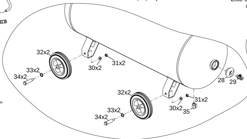
Figure 3 / Abbildung 3 / Рисунок 3 GK 500-3,0/200 Else see Figure 1 / Else siehe Abbildung 1 / Остальное смотри рисунок 1
