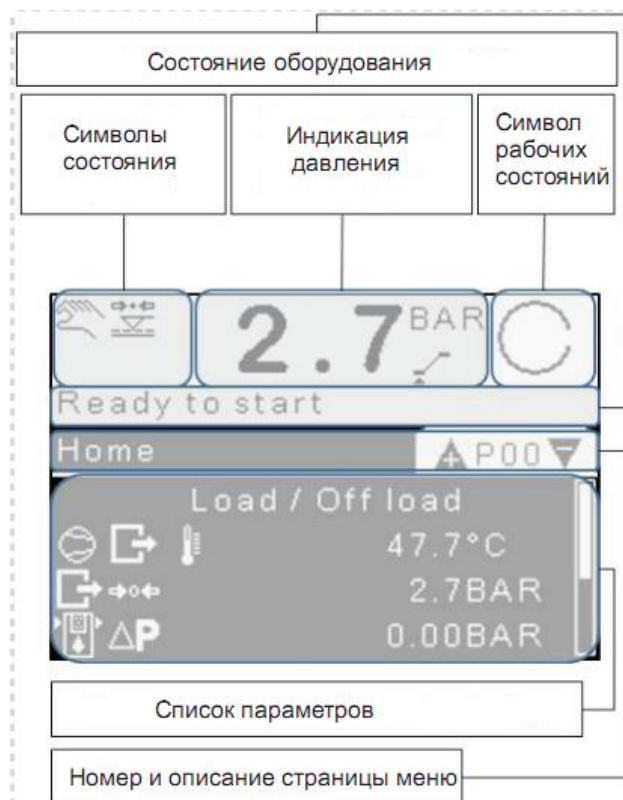
Рис. 1. Дисплей контроллера
